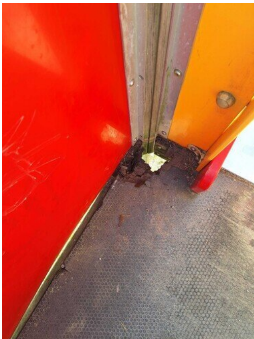
Kuva 41 Vaneri laho
