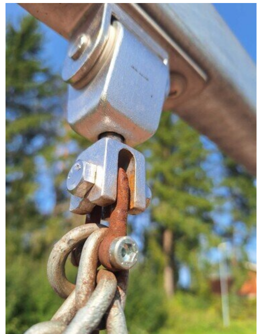
Kuva 14 Sakkelit ruosteessa/kuluneet
